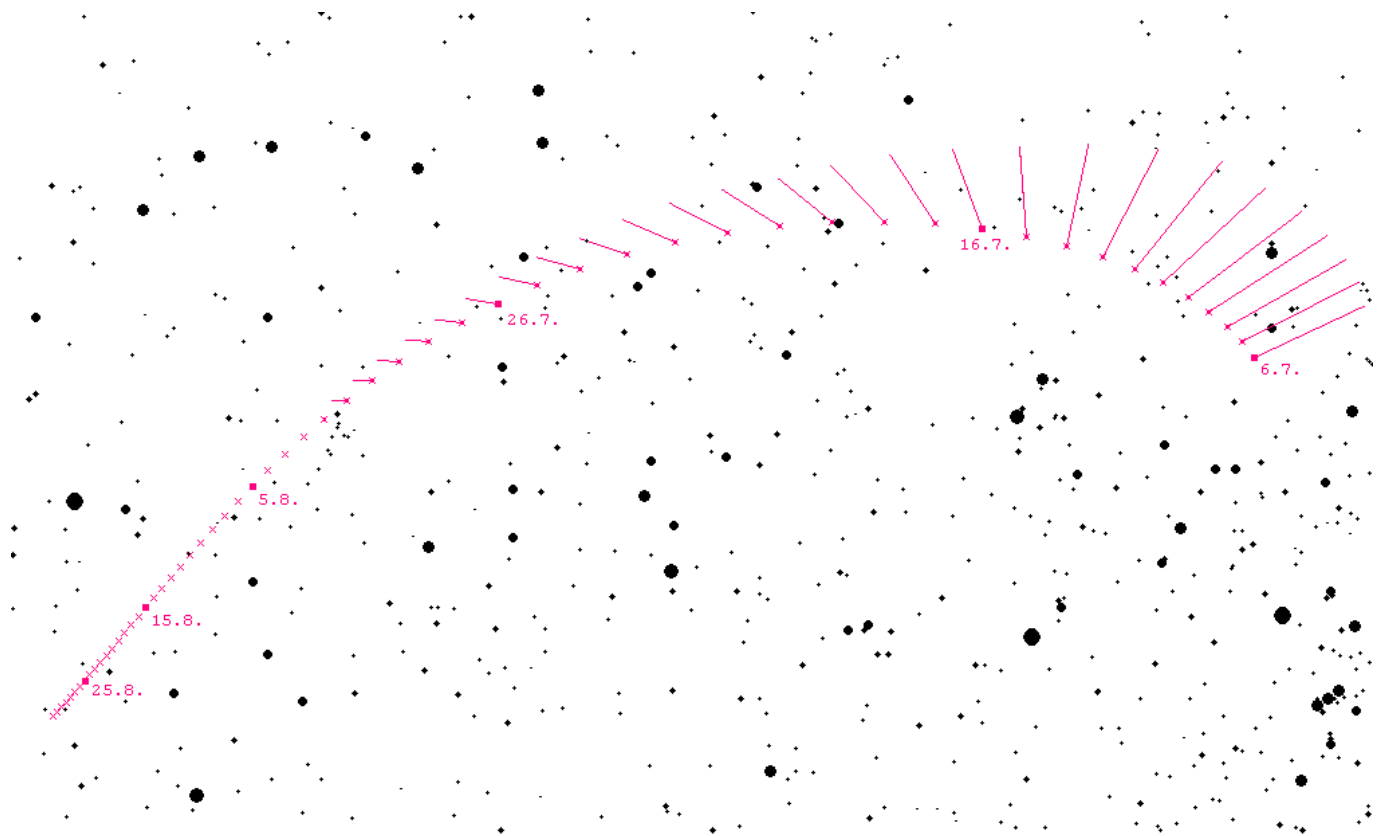
Bewegung des Kometen C/2020 F3 (NEOWISE) vom 6.7.20 bis 1.9.20
