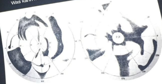
Karte Mädler-Beer 1840, 10 cm Teleskop
